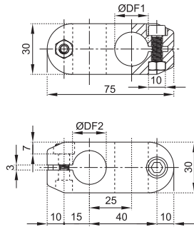
N202 大十字承夹 N202 CROSS CLAMP
