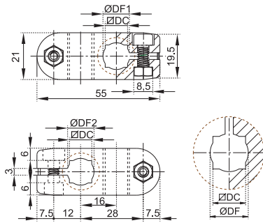
N201 小十字承夹 N201 CROSS CLAMP
