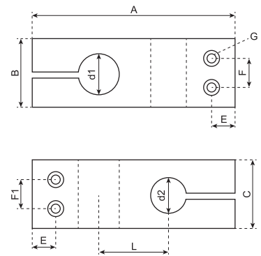
N200D 系列异径双孔十字夹 (双螺栓型) N200D UNEQUAL DIAMETER DOUBLE HOLE CROSS CLAMP (DOUBLE BOLT)
